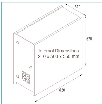
Caisson De Protection Pour UC 1 Ventilateur 210 x 500 x 550 (Intérieur)
